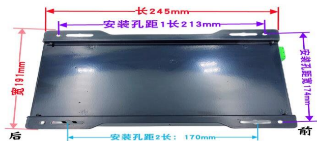
精创电源HJCH-1800W底部安装尺寸图
